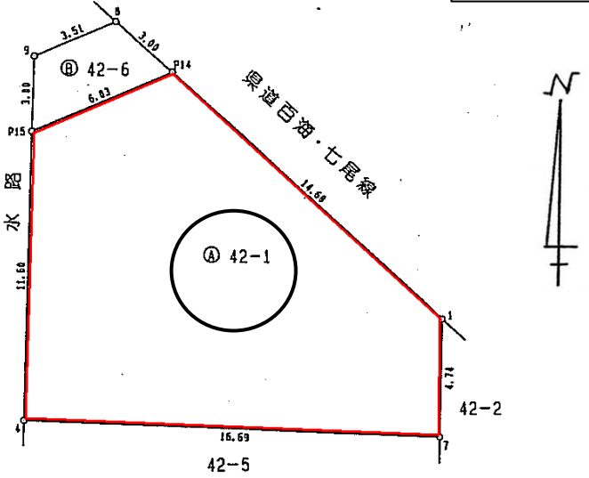
測量図
